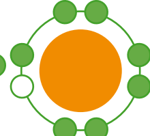
Molécule attaquée
